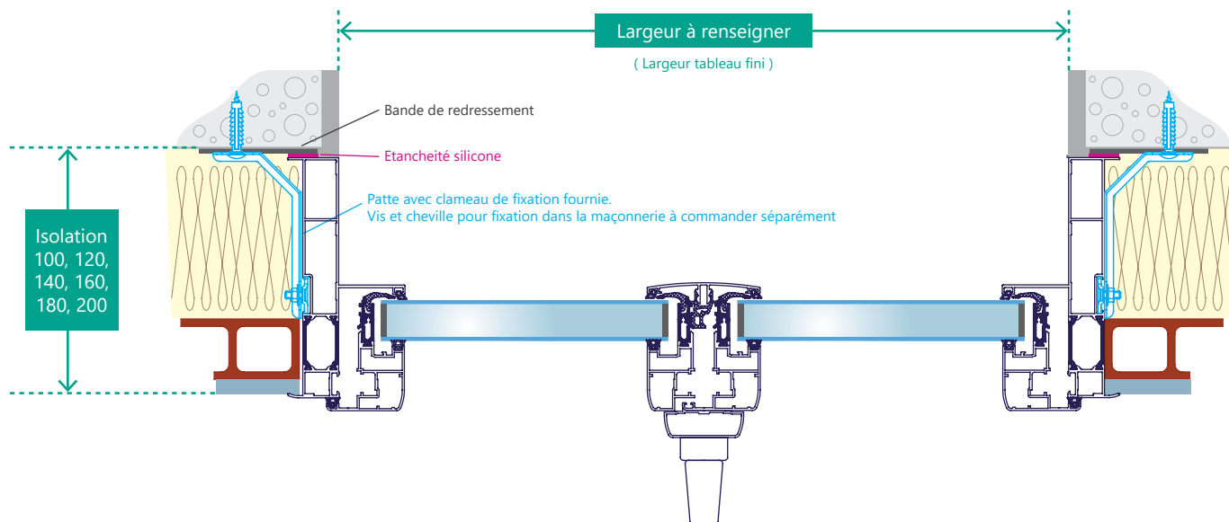
Fig 11. Coupe horizontale
