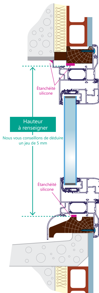
Fig 2. Coupe verticale
