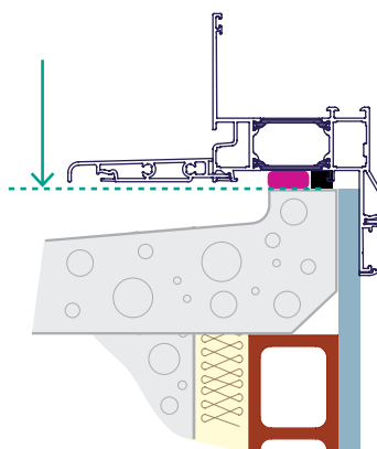
Fig 4. Variante avec suppression de l'appui en bois
