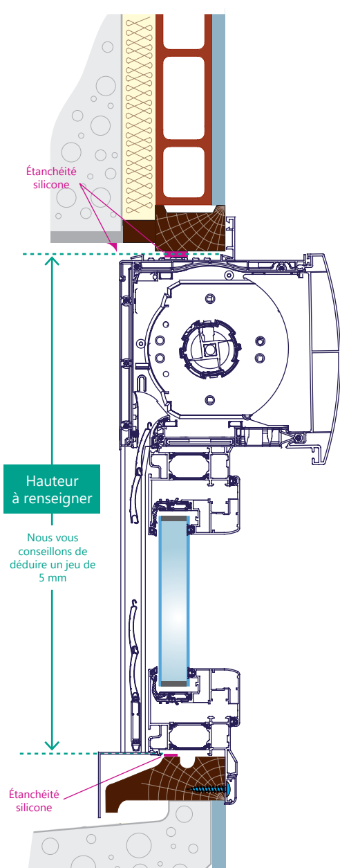
Fig 7. Coupe verticale conservation du dormant bois
