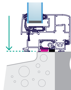
Fig 5. Variante avec seuil en aluminium
