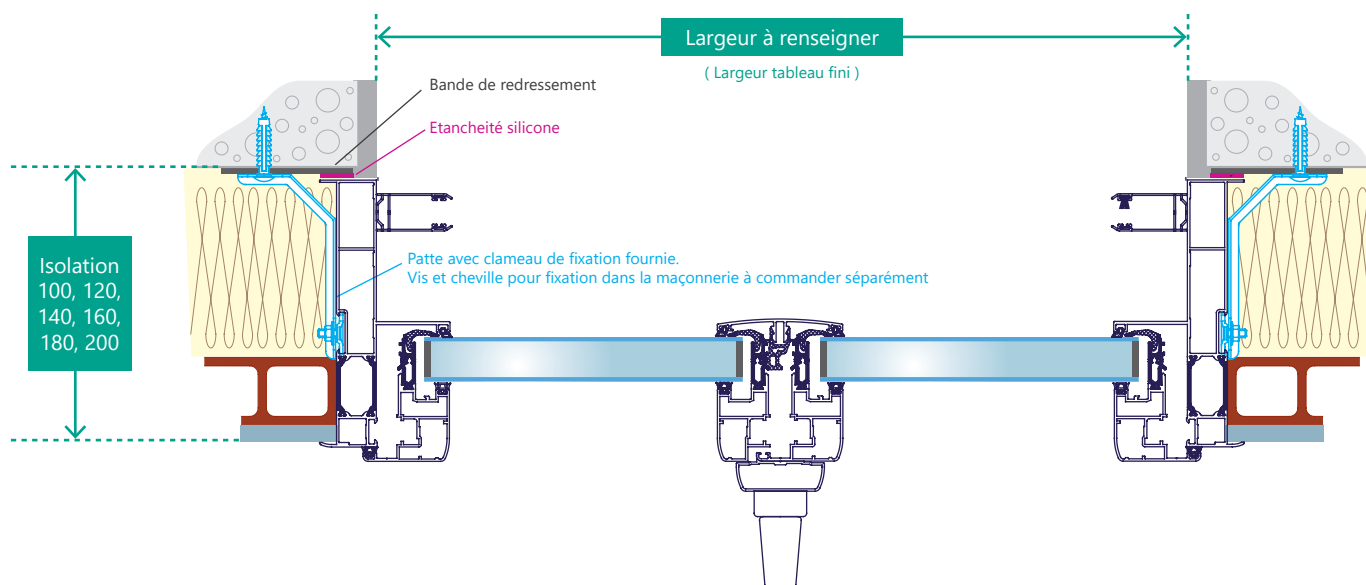
Fig 14. Coupe horizontale
