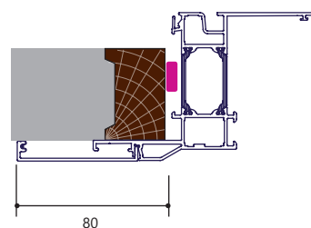
Fig 3. Moulure(s) intérieure(s) rapportée(s) (option)
