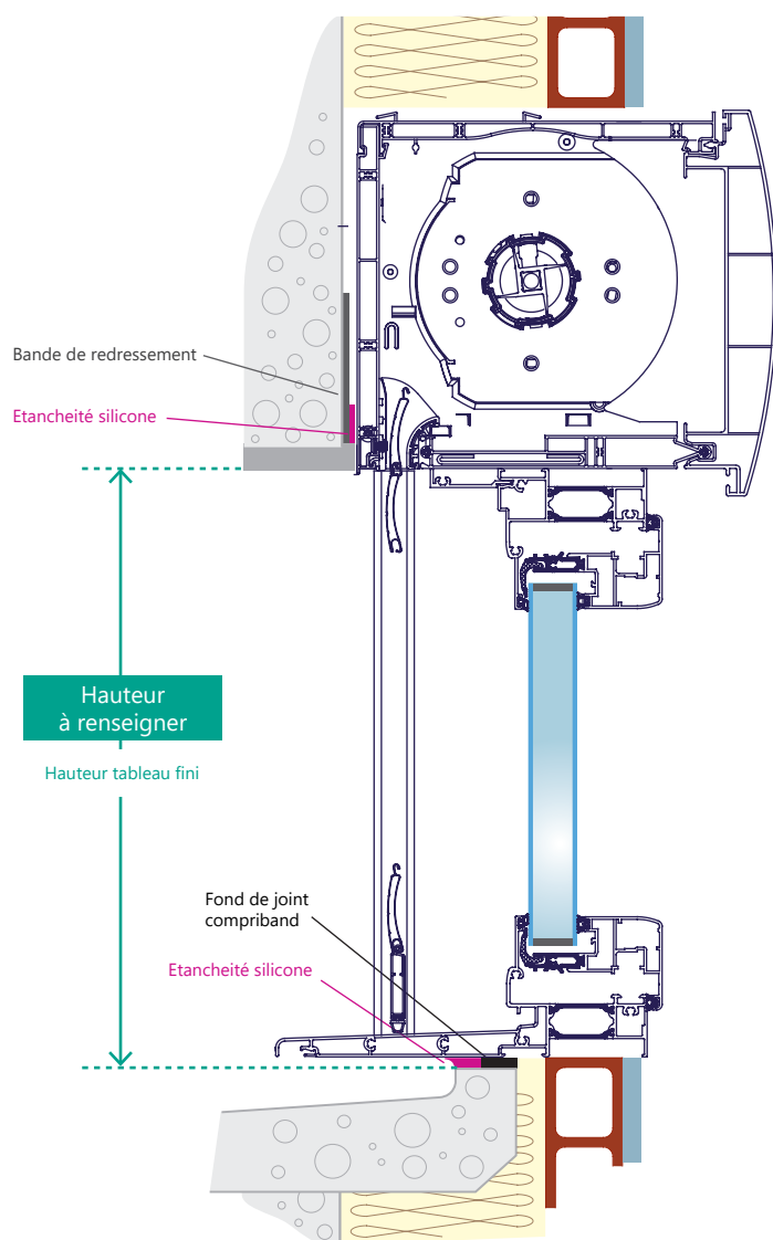
Fig 15. Coupe verticale
