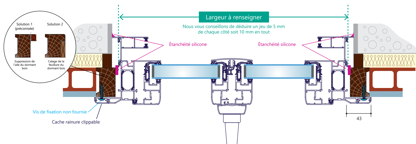
Fig 6. Coupe horizontale
