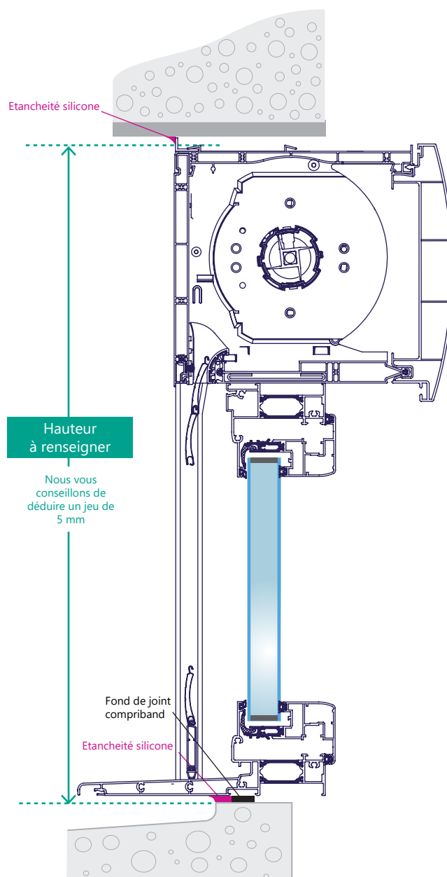
Fig 22. Coupe verticale avec volet roulant
