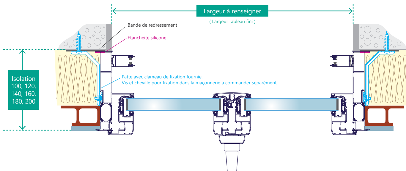
Fig 17. Coupe horizontale
