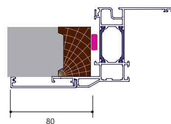
Fig 9. Moulure(s) intérieure(s) rapportée(s) (option)
