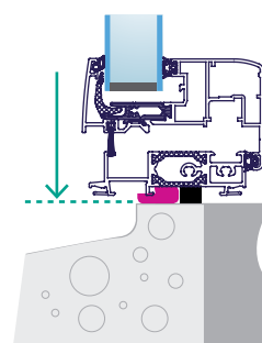
Fig 10. Variante avec seuil en aluminium
